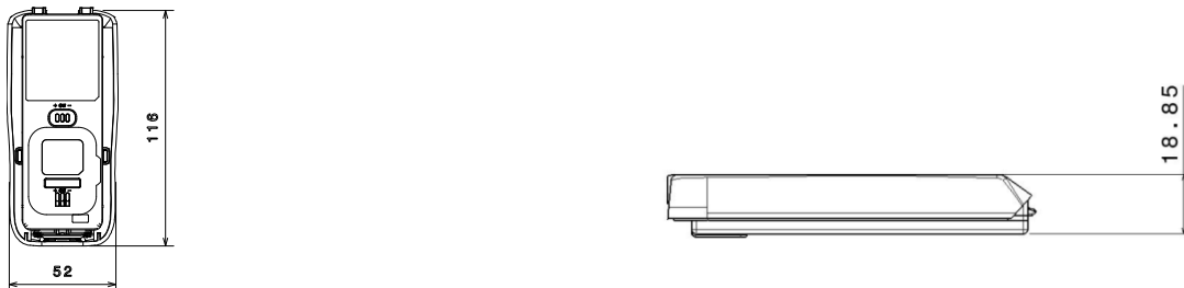
Obrázek: Základní rozměry baterie
